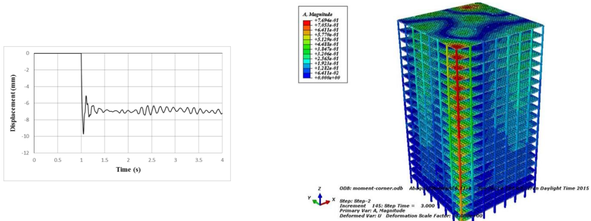
شکل ۱۱: تاریخچه جابجایی در گره بالای ستون حذف شده در حالت اول.
