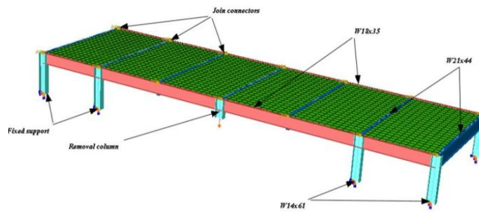
شکل ۴: جزئیات شرایط مرزی مدل صحت سنجی بر اساس [۱۳].
