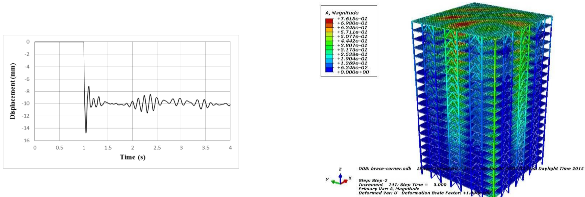
شکل ۱۹: تاریخچه جابجایی در گره بالای ستون حذف شده در حالت سوم.
