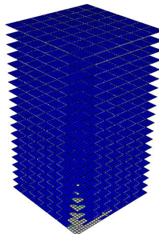
شکل ۳۲: خرابی فشاری بتن دال در حالت سوم.
